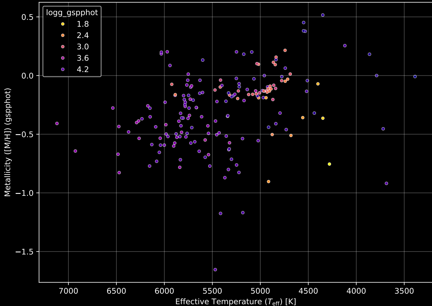
APOGEE DR17 Field: [289-33-O_TESS] Stellar Population Parameters (n= 182)
