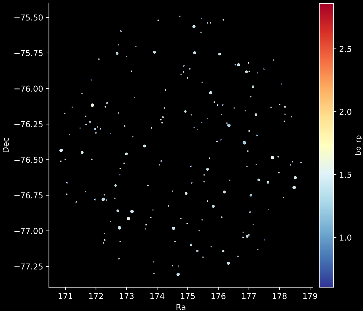
APOGEE DR17 Field: [289-33-O_TESS] Stars: 182
