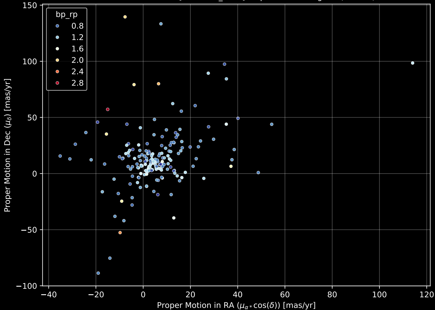
APOGEE DR17 Field: [289-33-O_TESS] Proper Motion Diagram (n= 182)
