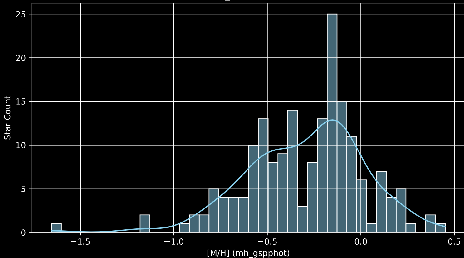
APOGEE DR17 Field: [289-33-O_TESS [M/H] (mh_gspphot) (n= 181)
